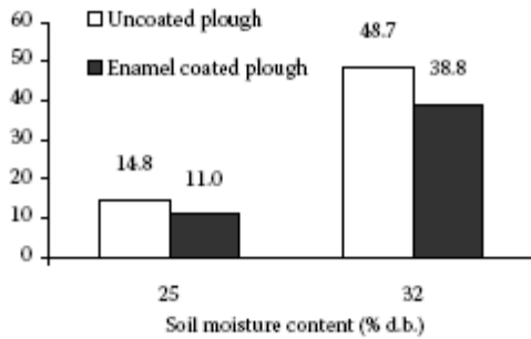
Fig. 2. Specific draught (kPa)
